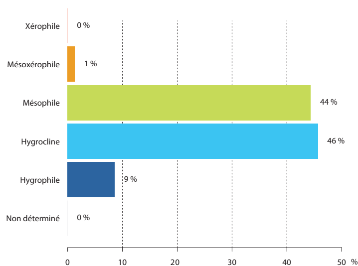
Niveau hydrique
