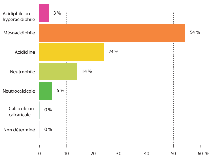
Niveau trophique
